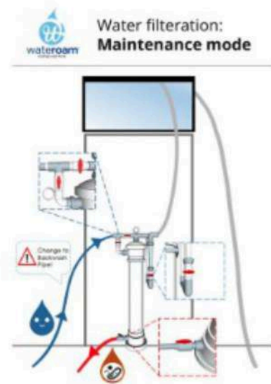
Fig. 3: Backflush
